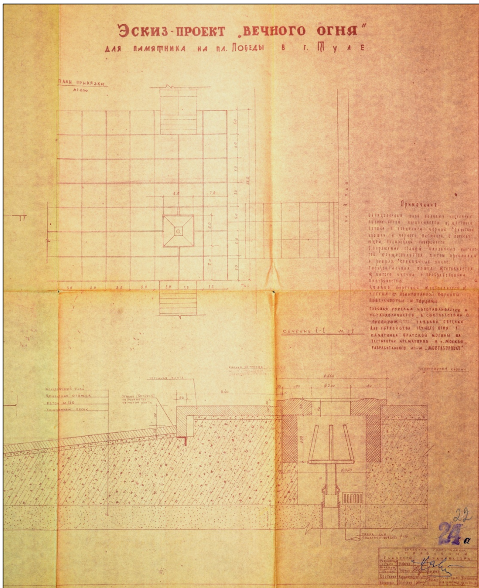
Рис. 5. Фрагменты эскиз-проекта «Вечного огня» для памятника на площади Победы в г. Туле. С подписью главного архитектора Тулы Назарова [18, л. 22]
